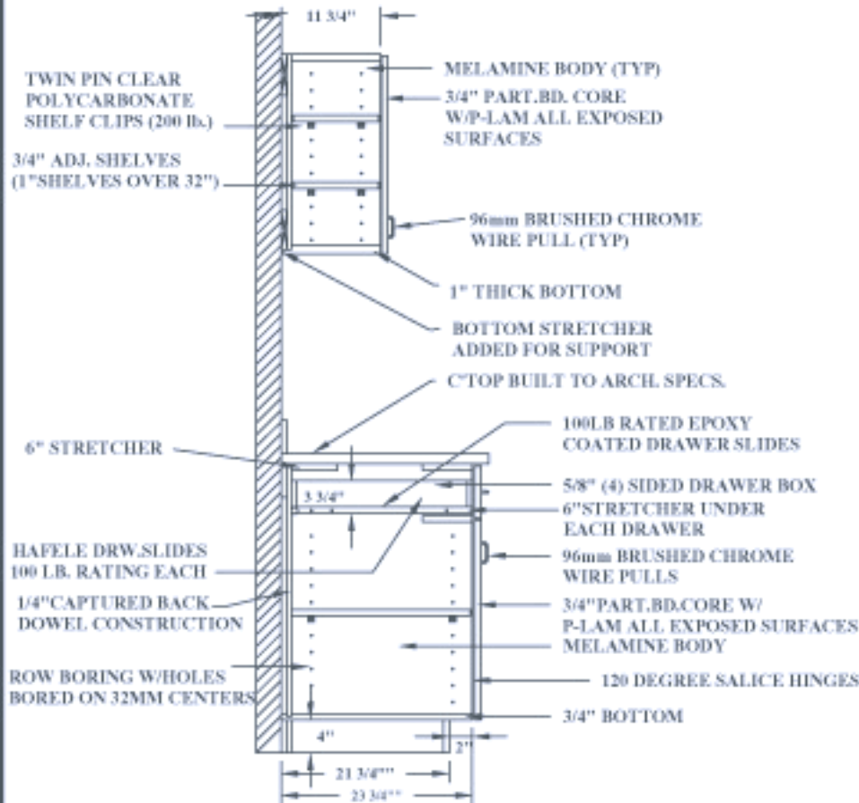
TYP. BASE DOOR/DRW. & WALL CABINET
