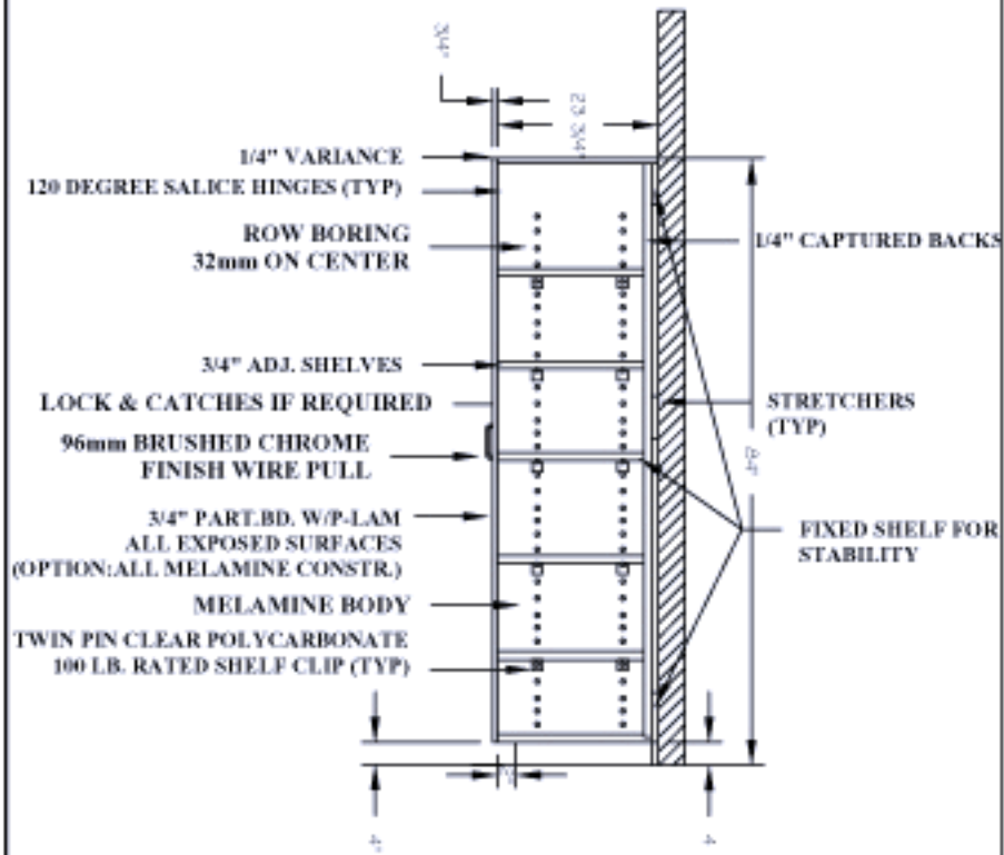
LEFT SIDE
